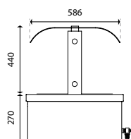
Glasopbouw tweezijdig afgerond
