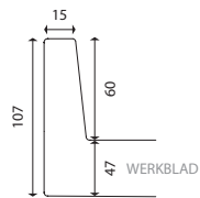
Opstaande rand
