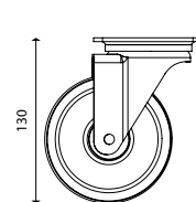
Zwenkwiel
